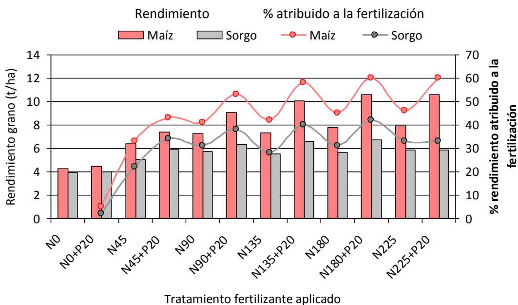
Figura 3. Efecto del nitrógeno y el fósforo en maíz en regadío y sorgo (media durante 40 años). Se aplicaron tratamientos de nitrógeno de 0, 20, 45, 90, 180 y 225 kg/ha sin y con aplicación de fósforo (20 kg/ha). Fuente: Stewart et al. , 2005.
