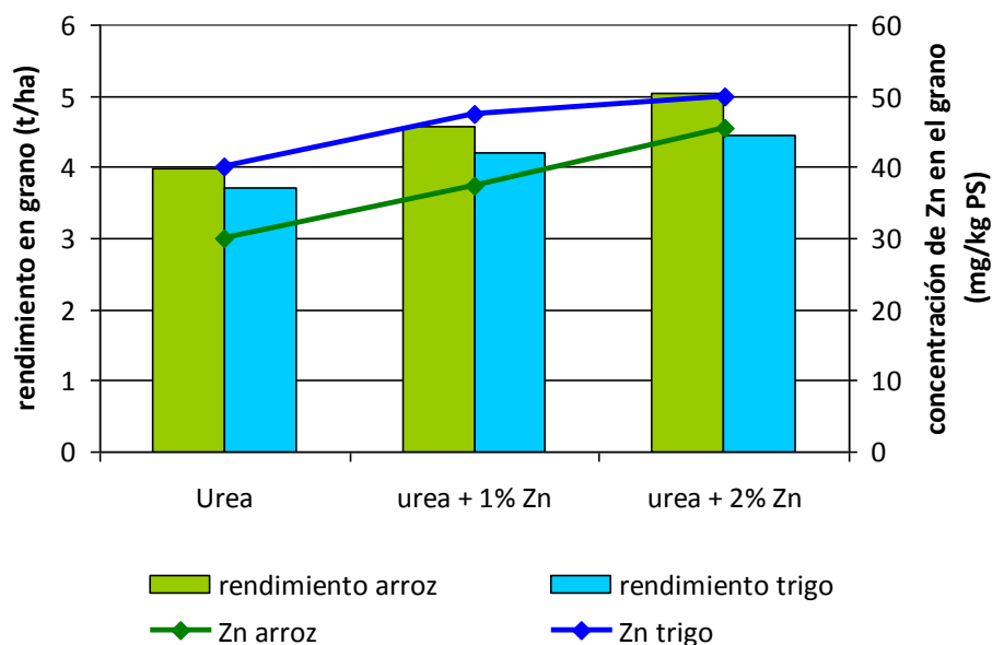
Figura 5. Rendimiento y contenido de Zn del grano de arroz y trigo dependiendo de las aplicaciones de urea enriquecidas con Zn en el campo experimental de IARI, Nueva Delhi (India). Fuente: Shivay et al. , 2008 en IPNI/IFA 2012.
